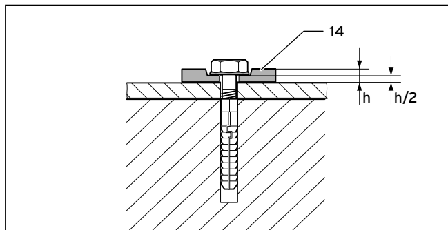
8.27 Upevnění s pružnými podložkami
