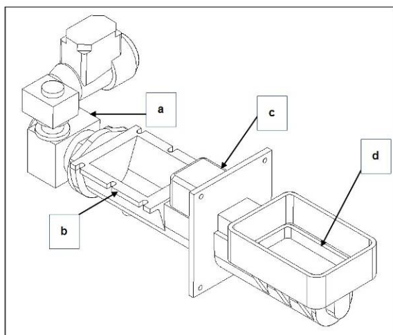
Obr. 2 Konstruktivní uspořádání hořáku
