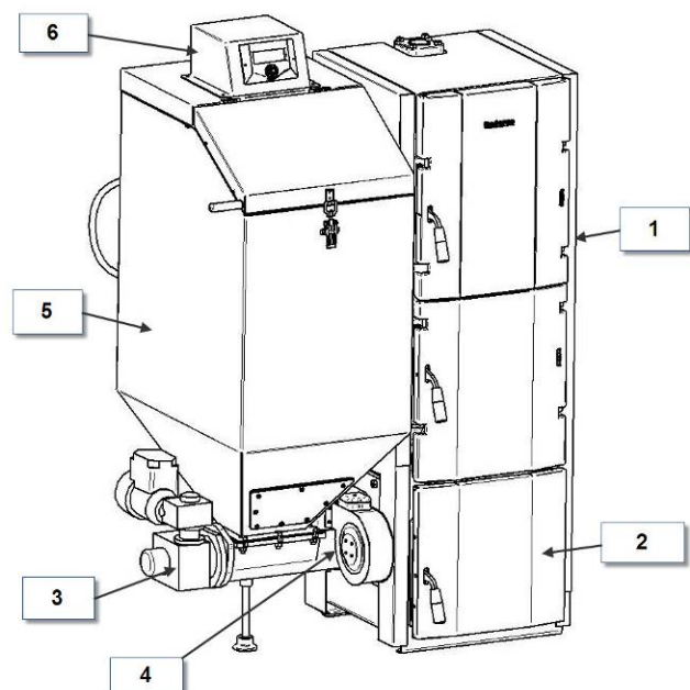
Obr. 1 Konstrukční uspořádání
