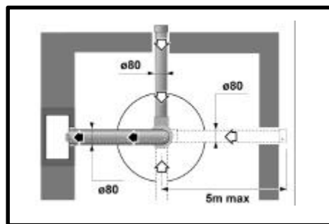
Obr. 6: Sada na oddelený prívod vzduchu a odtah spalín - maximální délky při vyústění na fasádu:
