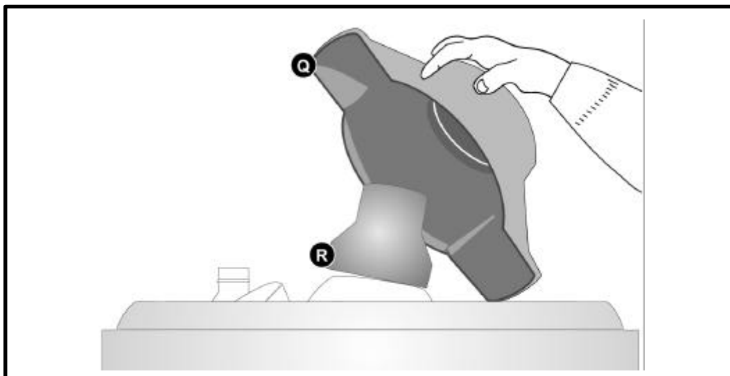
Obr. 8: Sada na oddelený prívod vzduchu a odtah spalín - postup při montáži Q - Plastový kryt R - Hliníková redukce
