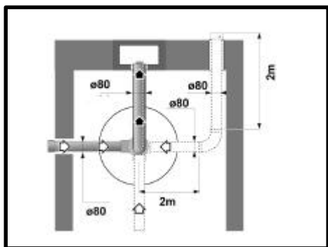
Obr. 6: Sada na oddelený prívod vzduchu a odtah spalín - maximální délky při vyústění na fasádu:
