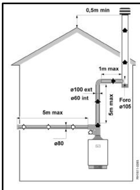
Obr. 7: Sada na oddelený prívod vzduchu a odtah spalín - maximální délky při odvodu spalín spalínovou šachtou.
