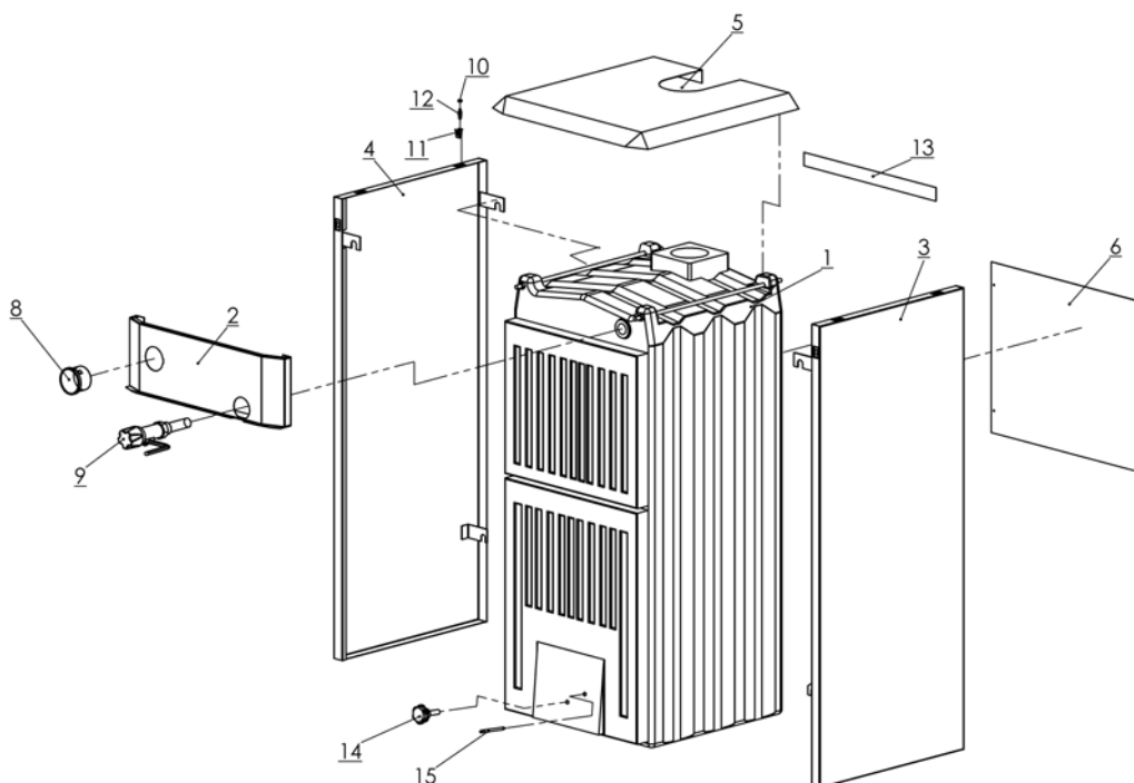
obr. 4: Montáž opláštění
