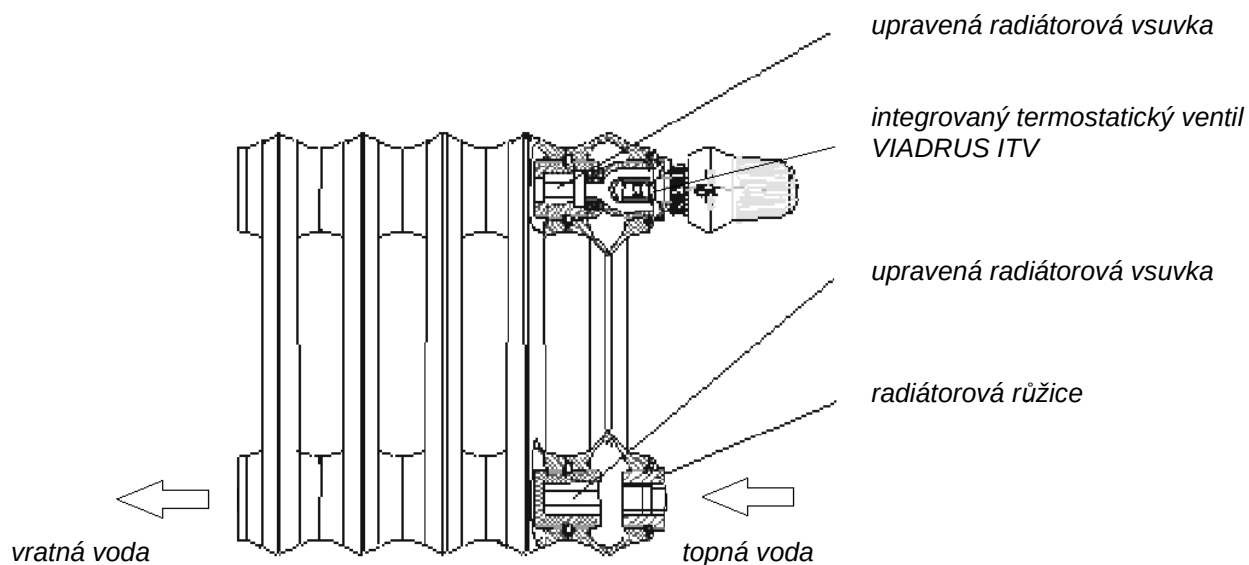
Obr. č. 2 Příklad nové instalace s integrovaným termostatickým ventilem (boční připojení)
