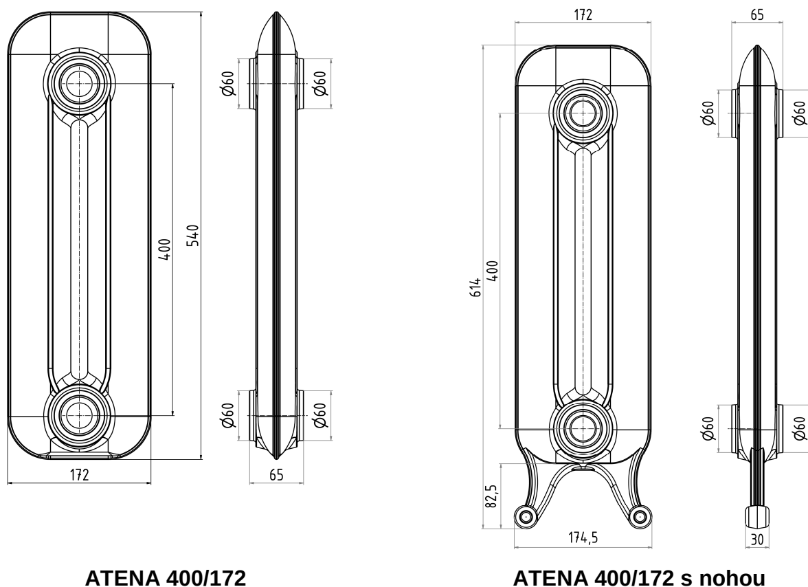
Obr. č. 2 Hlavní rozměry článků ATENA
