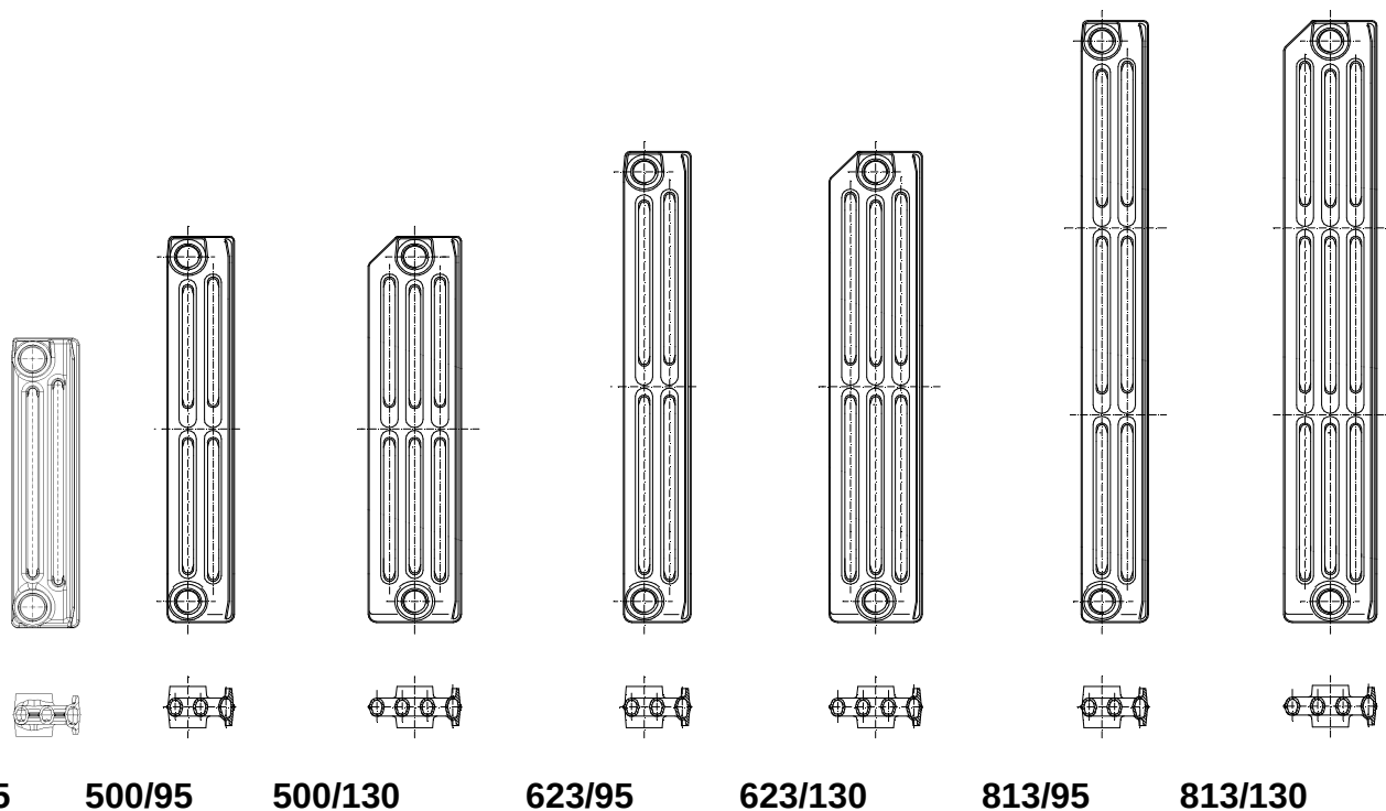
Obr. č. 1 Otopné články typu Termo
