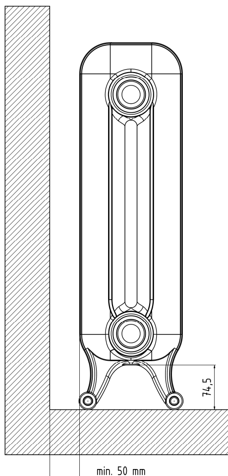
Obr. č. 3 Osazování otopných těles ATENA
