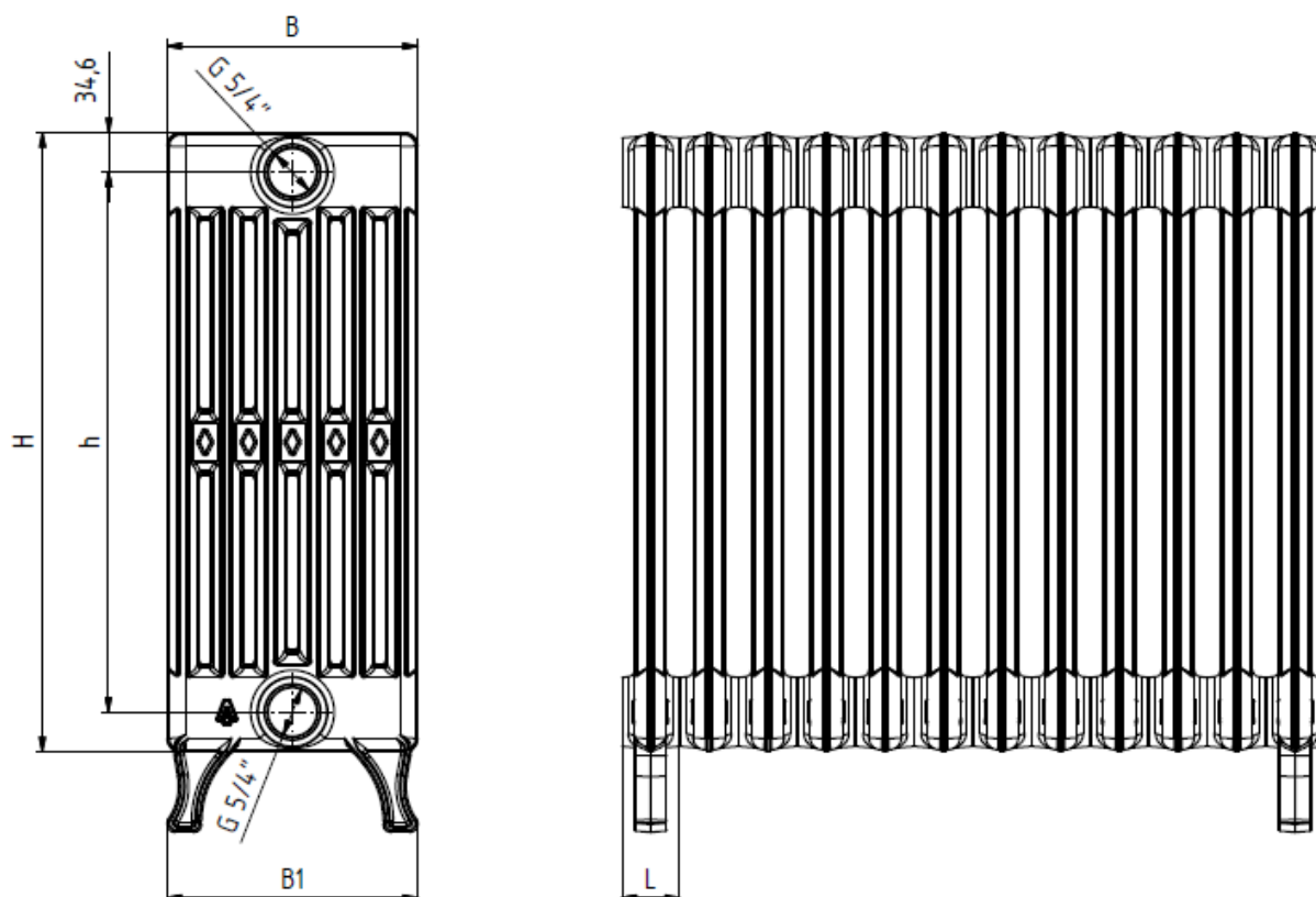
Obr. č. 2 Hlavní rozměry článků HELLAS
