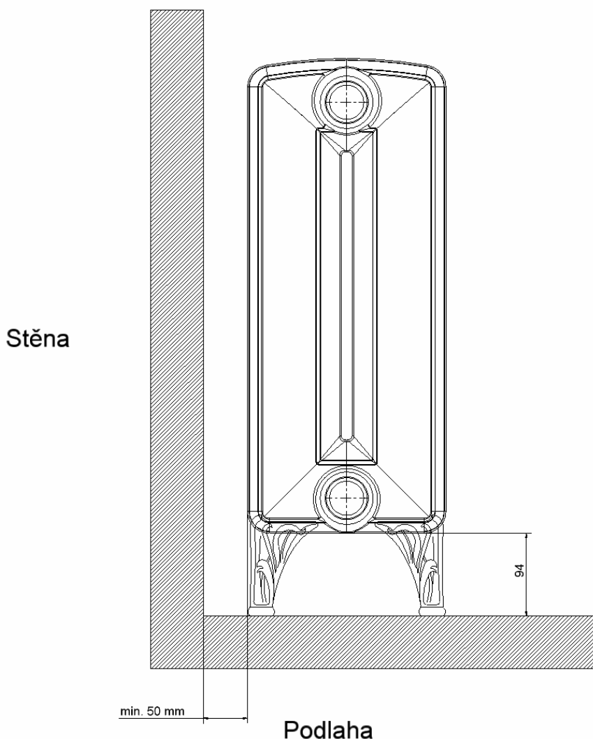
Obr. č. 3 Osazování otopných těles BOHEMIA R
