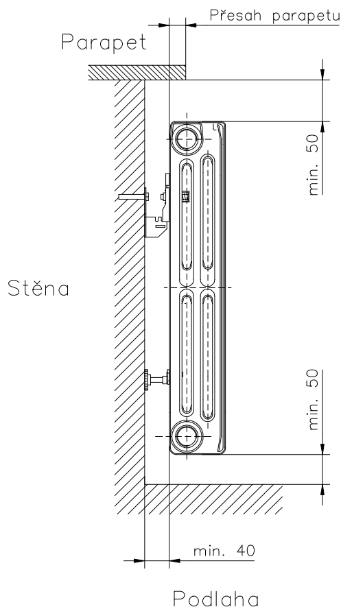
Obr. č. 3 Osazování otopných těles Termo
