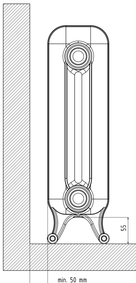
Obr. č. 3 Osazování otopných těles WINDSOR
