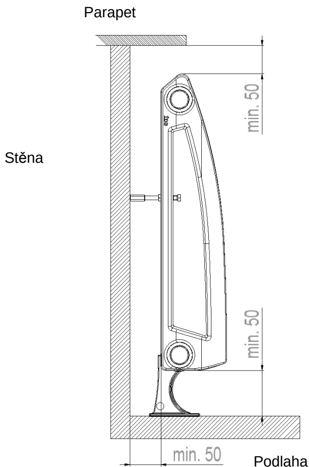
Obr. č. 3 Osazování otopných těles STYL
