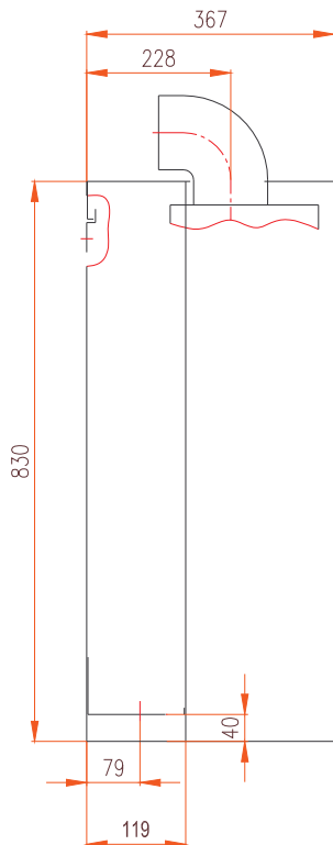
ŘEZ I-I
