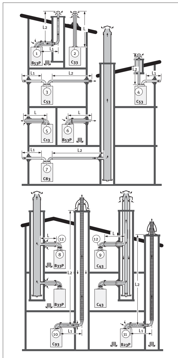
Použitelný přívod vzduchu/odvod spalin
